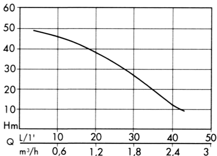
SUB 6S raksturlīkne
