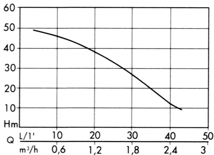
Dominator 4''-55/50 raksturliktne
