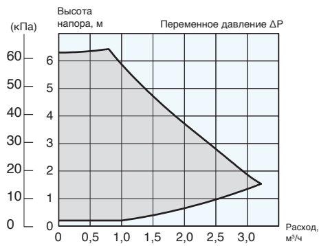
Технические характеристики циркуляционного насоса WILO YONOS PARA 25/6 гидравлических модулей EA 143/144
