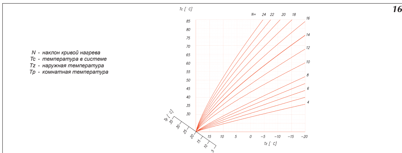
Рис.16 Кривая нагрева
