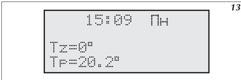
Рис.13 Общий обзор при конфигурации „ОТ. HET ВОД. HET” (выключен обогрев отопительной системы и контур обогрева бойлера)
