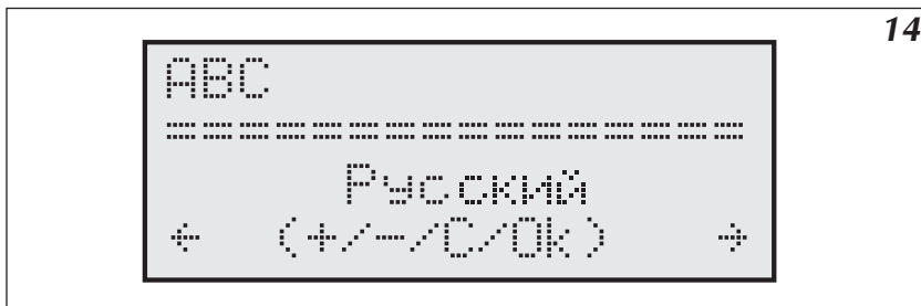
Рис. 14 Выбор языка
