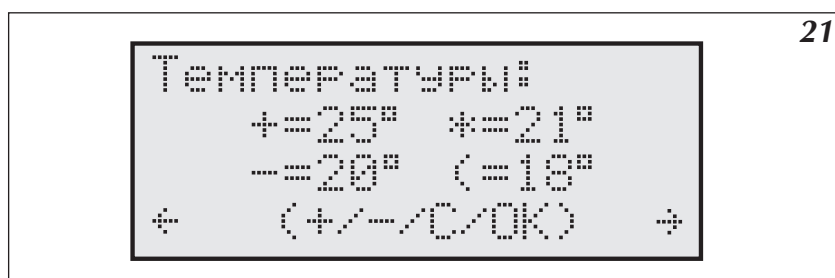
Рис.21 Страница установки суточных температур
