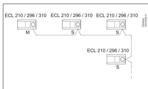
Vedējsekotājsistēmas savienojumi
