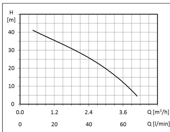
Sūkņa darba līkne
