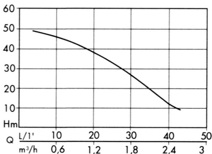
SUB 6S Plus raksturlīkne
