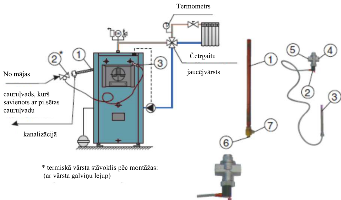
7. att. katla ECO CK 20-110kW termoizsardzības montāžas shēma slēgtā apkures sistēmā
