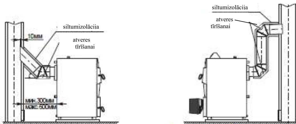
Iespējamā katla ECO CK pievienošana dūmvadam. (cietais kurināmais)
