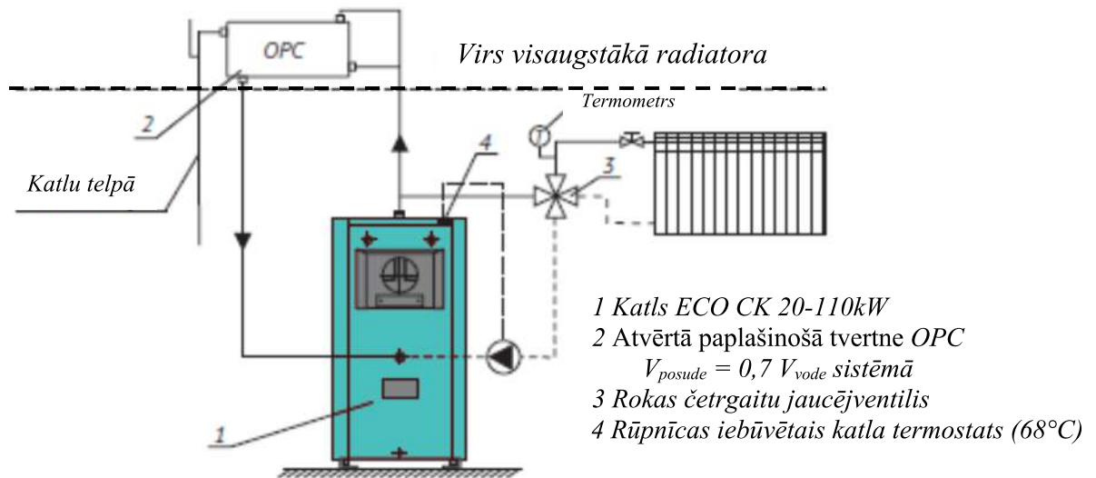
8. att. Katla pieslēgšanas atvērta apkures sistēmai principiālā shēma
