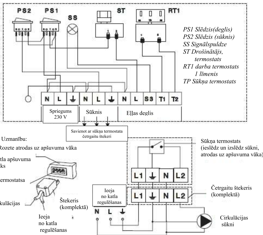
13. att. Katla ECO CK 20-110kW un sūkņa termostatsa regulēšanas elektriskā shēma, strādājot ar šķidro kurināmo/gāzi
