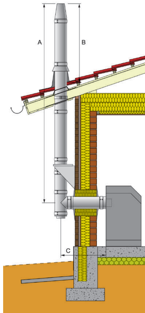
ICS25 moduldūmvada savienošana ar apkures iekārtu. Zīmējums ir ilustratīvs.
