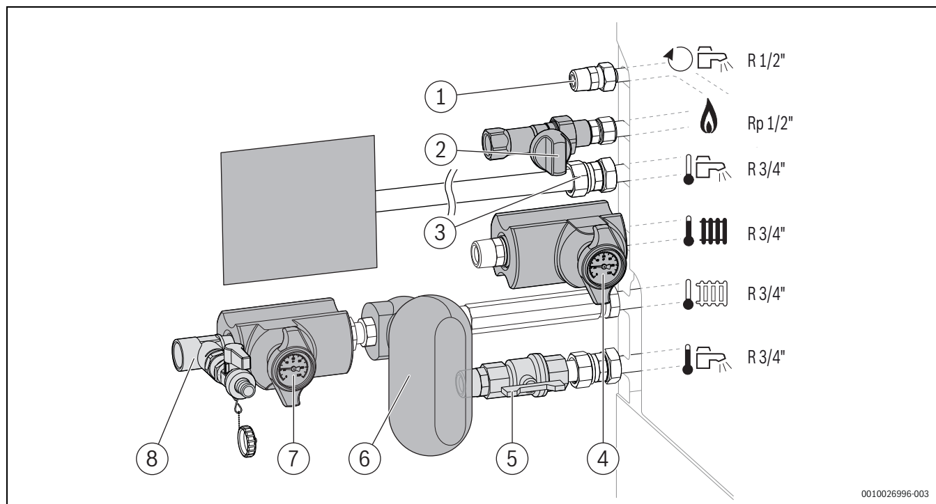
Att. 11 Piemērs: gāzes un ūdens puses pieslēgums ar krānu pieslēgšanas komplektu (piederums CS 28-1) kreisajā pusē
