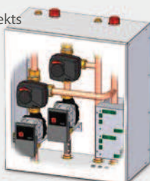
Hidraulikas komplekts
