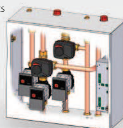
Hidraulikas komplekts
