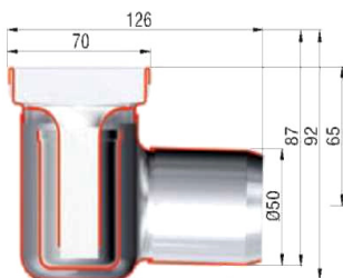
92 mm kanāls bez atloka
