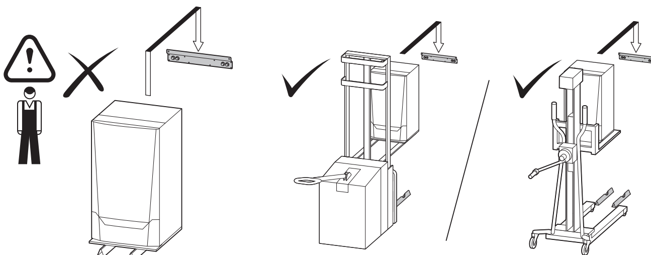
attēls6 Celšanas palīglīdzekļi
