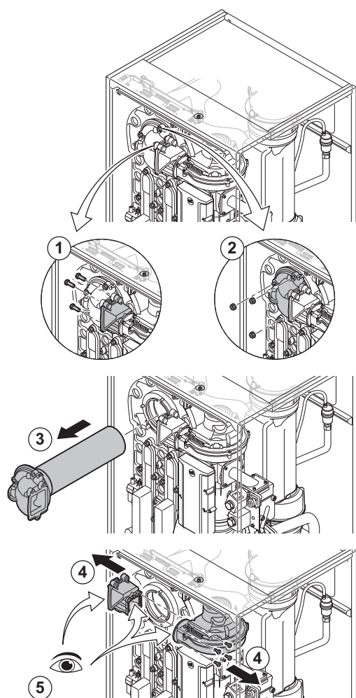
attēls75 Vienvirziena vārsta pārbaudīšana
