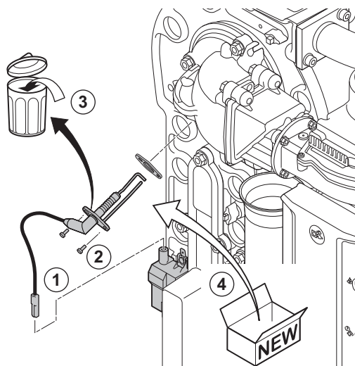
attēls74 Jonizācijas/aizdedzes elektroda nomaiņšana
