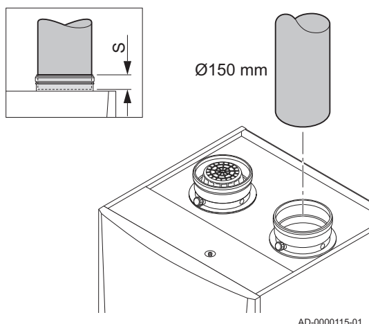
attēls20 Dūmgāzu izplūdes atveres pievienošana
