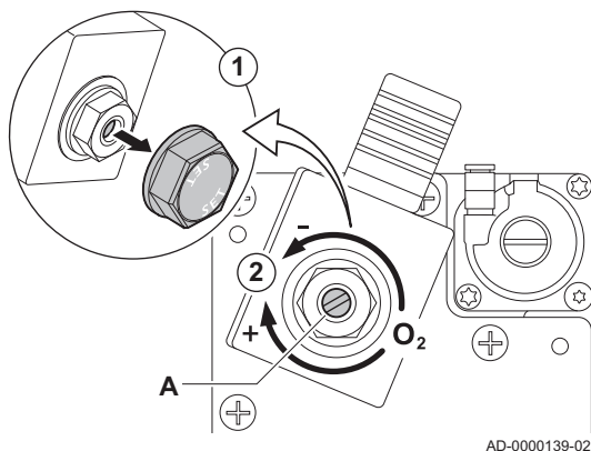
attēls43 Regulēšanas skrūves A pozīcija
