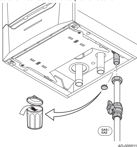
attēls15 Gāzes caurules pievienošana
