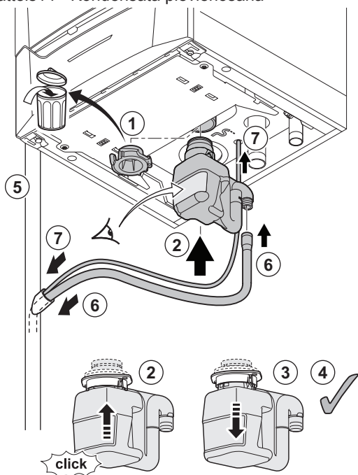
attēls14 Kondensāta pievienošana
