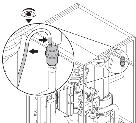
attēls70 Automātiskās vēdināšanas atveres pārbaudīšana
