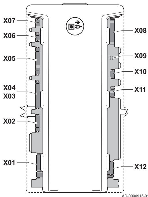
attēls22 Savienotāji no vadības bloka CU-GH06 (skats no priekšas)
