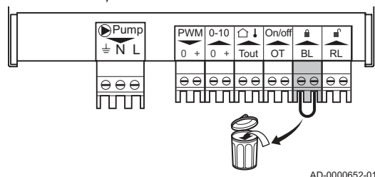
attēls35 Bloķēšanas ievade
