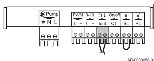
attēls29 Āra sensors
