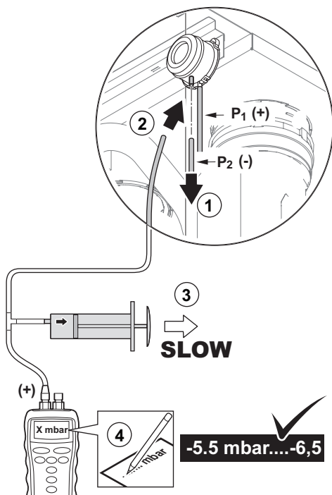
attēls69 Gaisa spiediena starpības slēdža - puse
