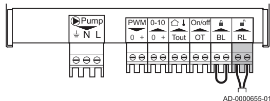
attēls36 Atvienošanas ievads
