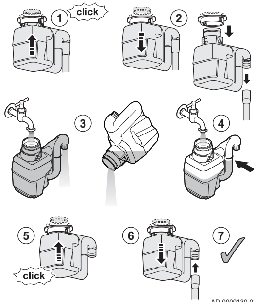
attēls73 Sifona tīrīšana
