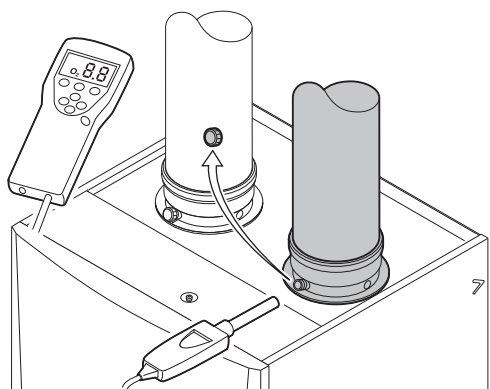
attēls40 Dūmgāzu mērpunkts
