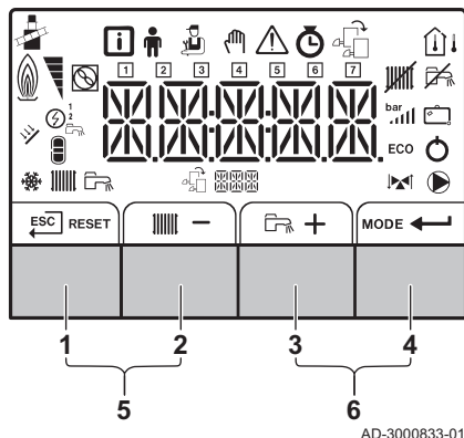
attēls5 Vadības panelis
