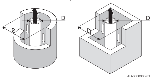
attēls16 Šahtas vai cauruļvada minimālie izmēri
