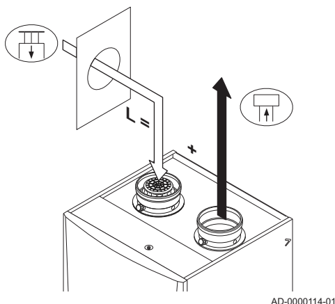
attēls19 Dažāda spiediena zonas
