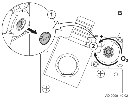
attēls45 Regulēšanas skrūves B pozīcija
