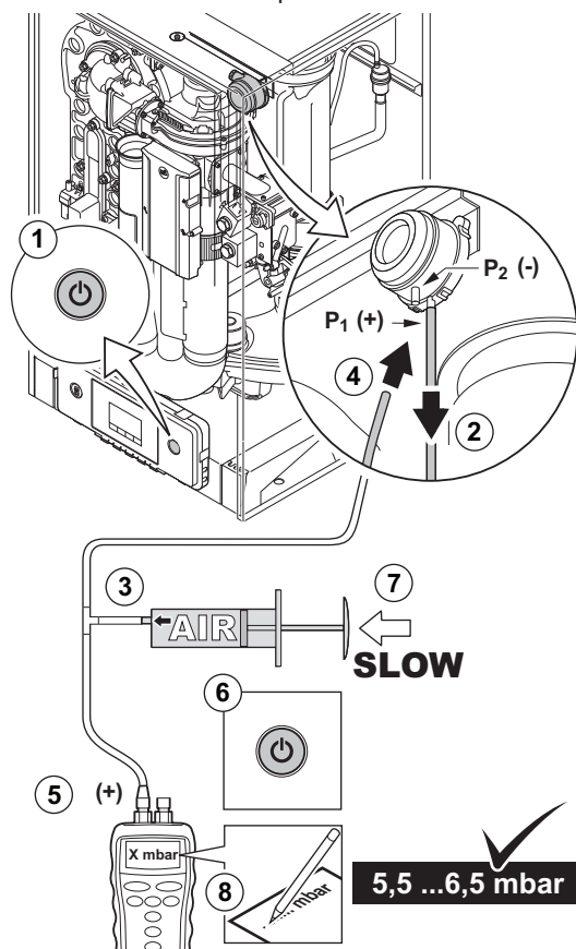
attēls68 Pārbaudiet gaisa spiediena starpības slēdža + pusi
