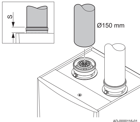
attēls21 Gaisa pievades pievienošana
