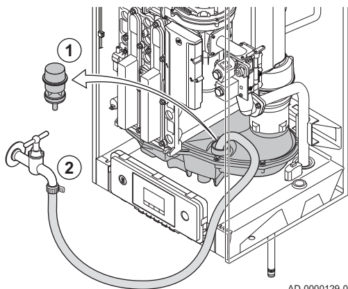
attēls72 Notīriet kondensāta kolektoru.
