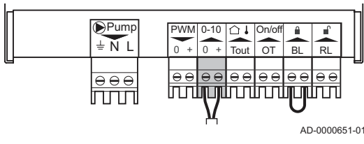
attēls33 Analogā ieeja
