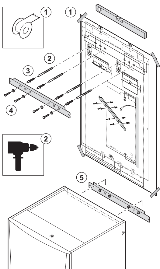
attēls11 Katla montāža
