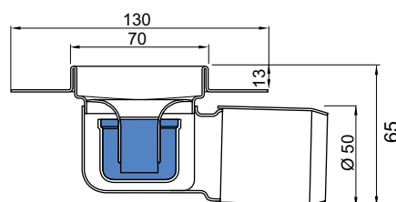
Pazemināts 65 mm kanāls ar atloku
