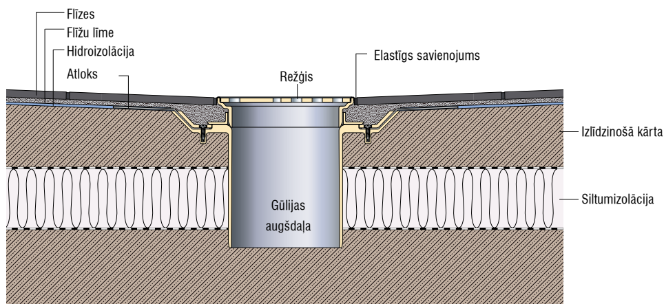
Gūlījas augšdaļa ar siltumizolāciju
