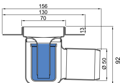
Standarta 92 mm kanāls ar atloku
