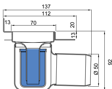
92 mm kanāls ar vertikālu atloku
