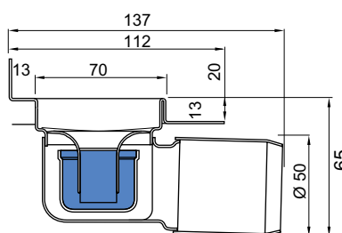
65 mm kanāls ar vertikālu atloku
