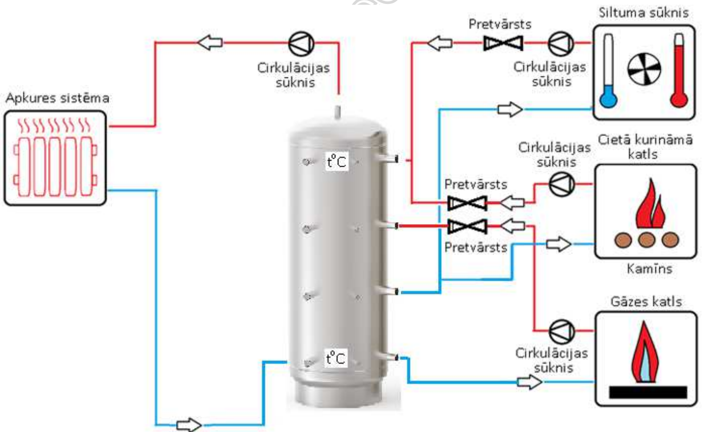
AT sērijas tvertnes darba principiālā shēma
