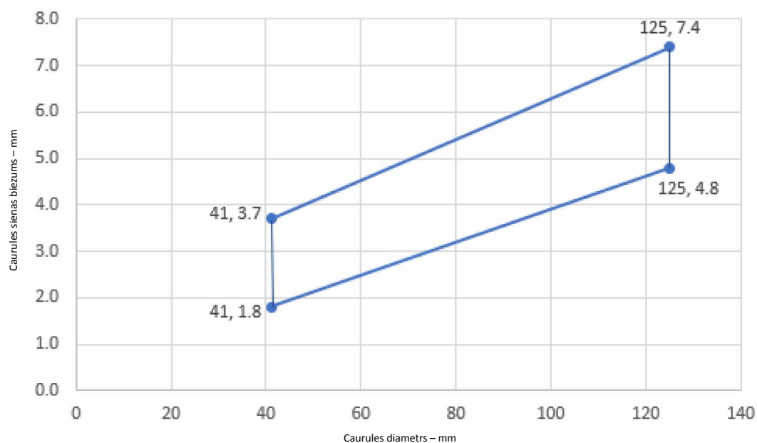
PVC-U caurules, diametrs 41–125 mm – EI 50 U/U
