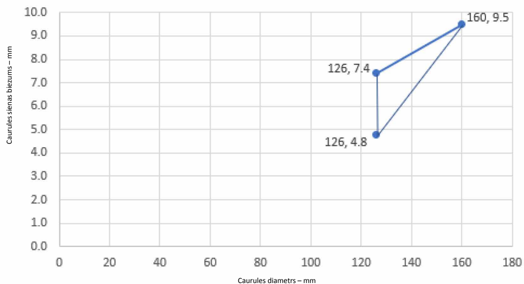
PVC-U caurules, diametrs 126–160 mm – E 120 U/U, EI 30 U/U
