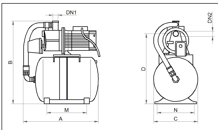
Габаритные размеры
