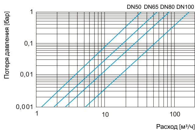
Графики потерь давления
