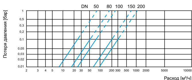
Графики потерь давления
