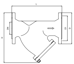
Размеры Y-Filter
