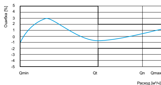
Типичная измерительная кривая
