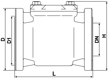
Размеры T-Filter
