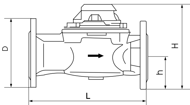
Размеры ЕТК-N-C
