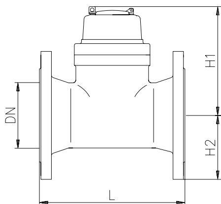
Размеры WI-N
