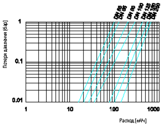
Потеря давления PN 10-4/ PN 16-4
