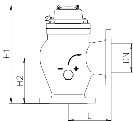
Размеры WB-N
