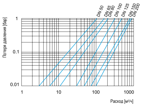
Потеря давления PN 10-5 / PN 16-5
