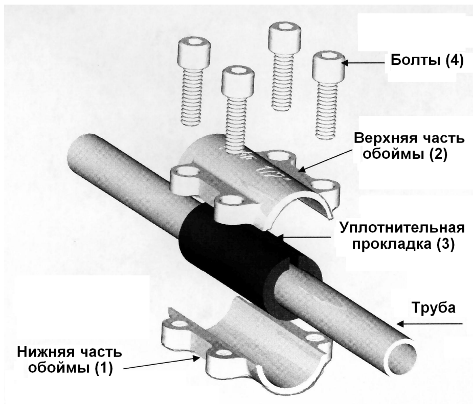
Ремонтная обойма DSK
