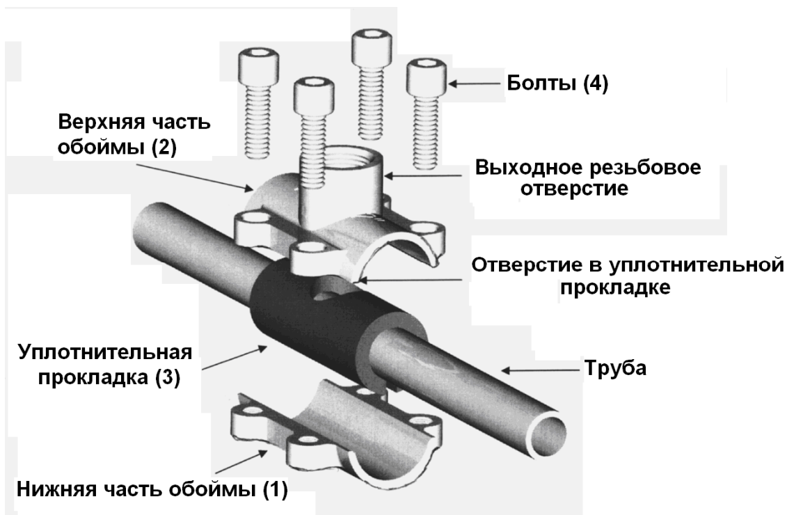
Ремонтно-монтажная обойма ANB
