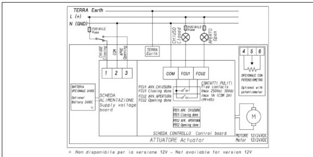
Att. 5 Piedziņas elektrosavienojumu shēma
