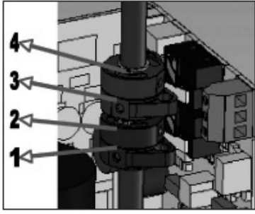
Att. 6 Ierobežojošo pārslēdzēju izcilņi
