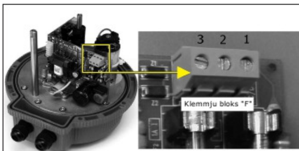
Att. 3 100-240 V modeļa panelis un klemmju „F” fragments
