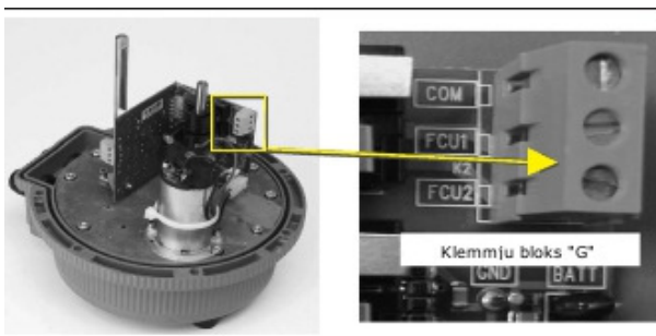
Att. 4 Kontroles panelis un klemmju bloka „G” fragments
