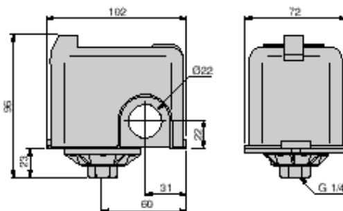
Spiediena slēdža FSG-2 izmēri:
